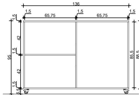
02 CORTE 02
